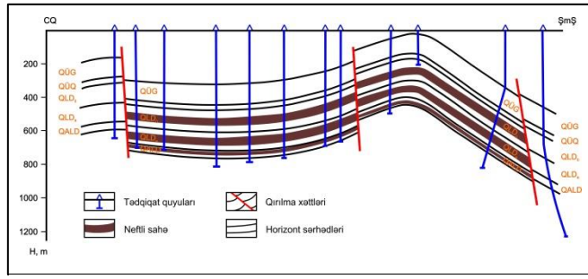
Şəkil 2. Pirallahı strukturunun şimal qırışıqlığına görə profil
