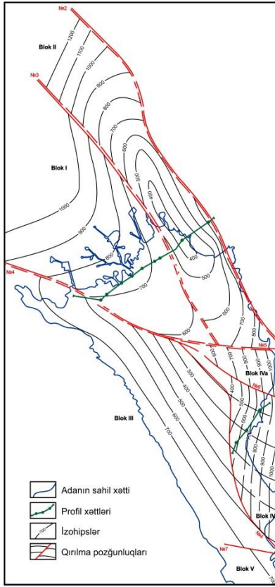
Şəkil 1. Pirallahı strukturunun QALD horizontunun tavanına görə struktur xəritəsi
