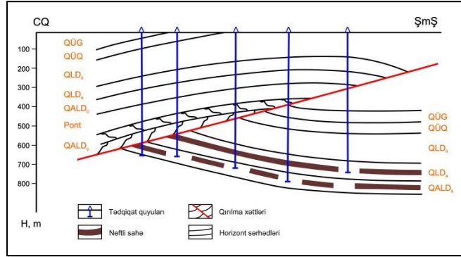
Şəkil 3. Pirallahı strukturunun cənub qırışıqlığına görə profil
